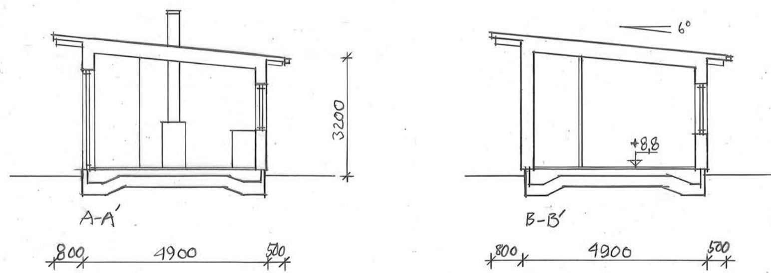
SEKTION A-A' OCH B-B'
